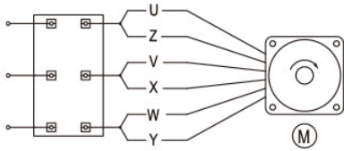
三相AC220V接线图 Three-phase AC220V Wiring Diagrams
