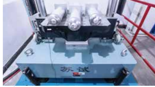
冲击试验台 / Shock Test Bench
